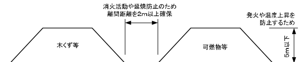
図表 3-24 可燃性廃棄物を並べて配置する場合
