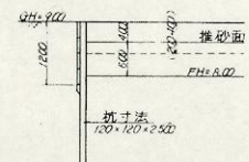
板 柵 断 面
