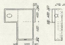
板 柵 断 面
