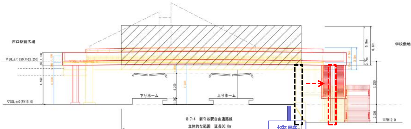
立面図①
