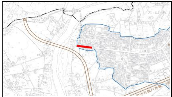
工事箇所 ⑧市道2025号線(松前台)
