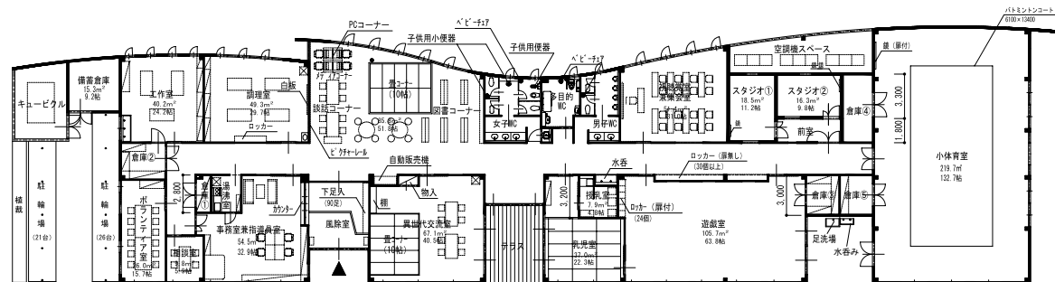
南守谷児童センター平面図
