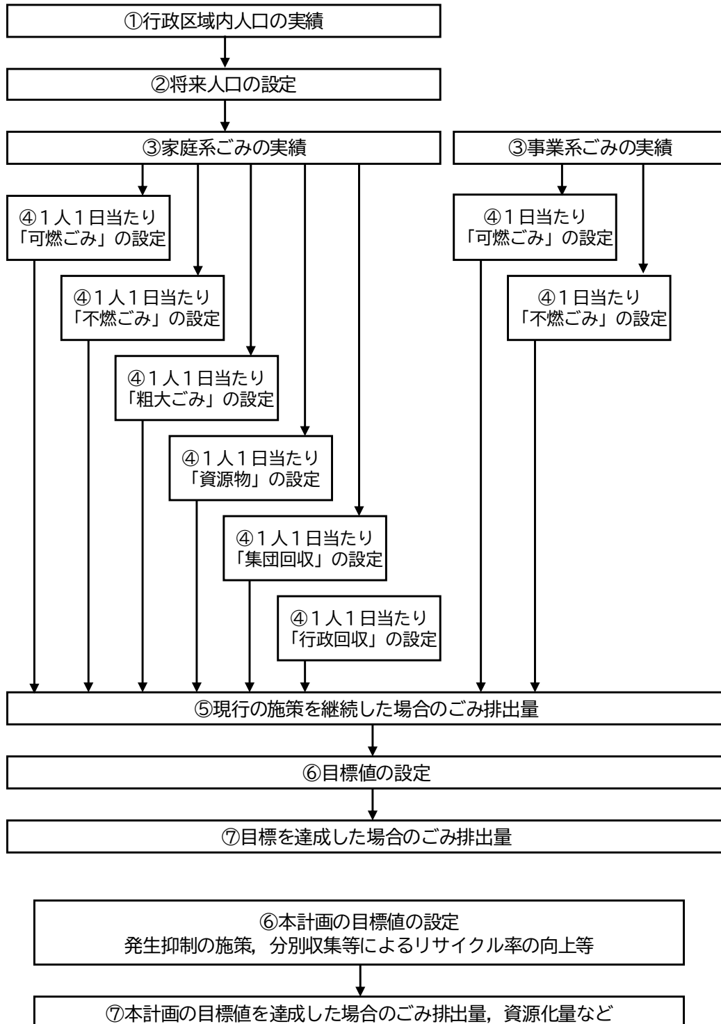
図 4-1 予測フロー
