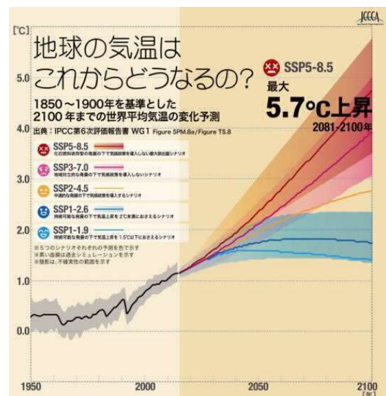
図 1-1 地球温暖化のメカニズムと 2100 年の気温予想
