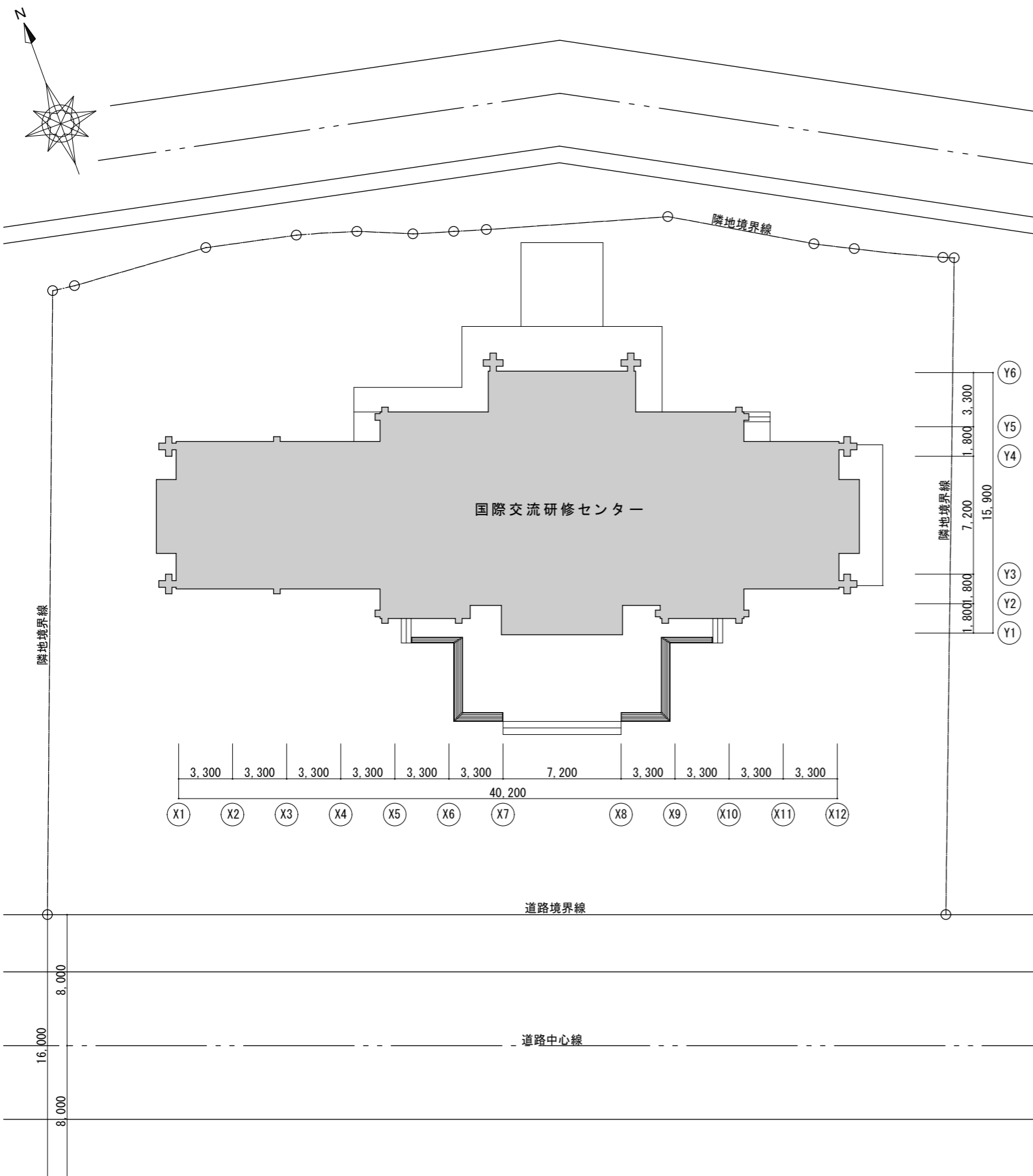
配置図 1/300
