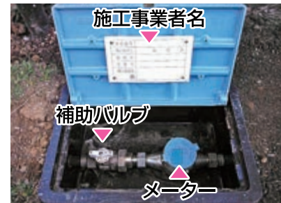
2 メーターボックスのふたを開けてメーターのパイロット（銀色の羽根車）の動きを見る。
